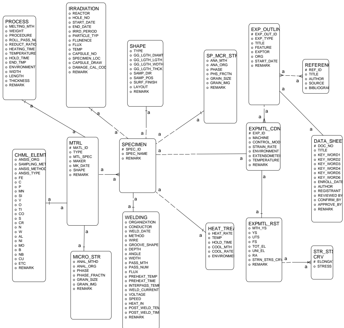
Fig. 1. 인장특성 DB의 ERD(Entry Relationship Diagram).
