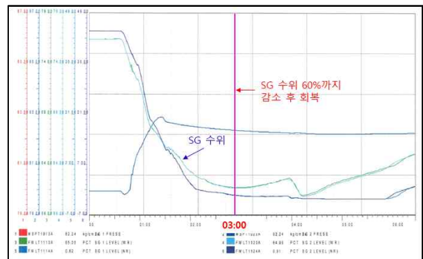
Fig. 2. CASE B : RPCS Manual actuation
